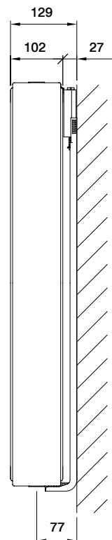
Rozmístění montážních otvorů Typ 11/20-22
