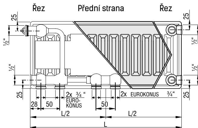
Radiátor s ventilem na levé straně
