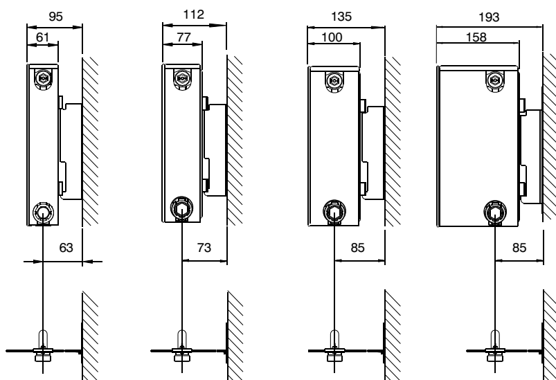
Montáž - delší bok L konzoly
